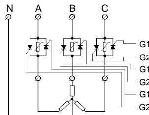
图 10: C4、K6 型应用 三相四线制移相触发
