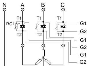
图 9: C4、K6 型应用 三相四线制移相触发
