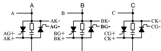
图 15: C8 全控型应用。单硅反并联, Y/ \Delta 接法。自动适应相序。
