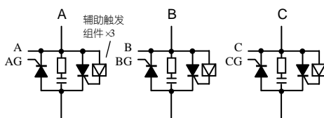
图 14: C7 型应用。单硅反并联, Y/ \Delta 接法。自动适应相序。 如果采用单硅和二极管反并联, 则不按图中三个辅助组件
