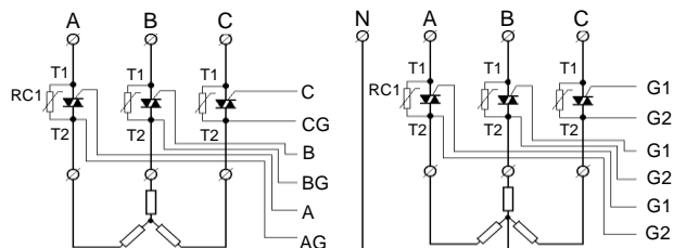
图 8: C5、K6 型应用 三相三线制移相触发
